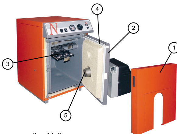
Рис. 14: Детали котла
